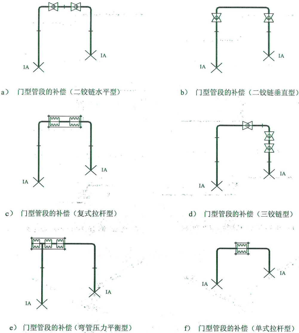
图 A.4 II型管道的补偿方式
