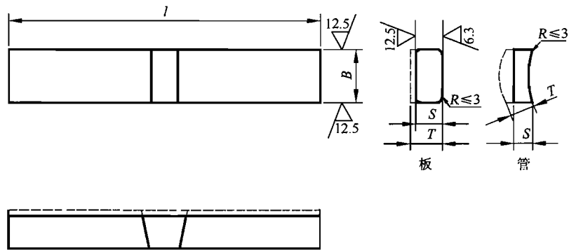
a) 板状和管状试件的面弯试样
