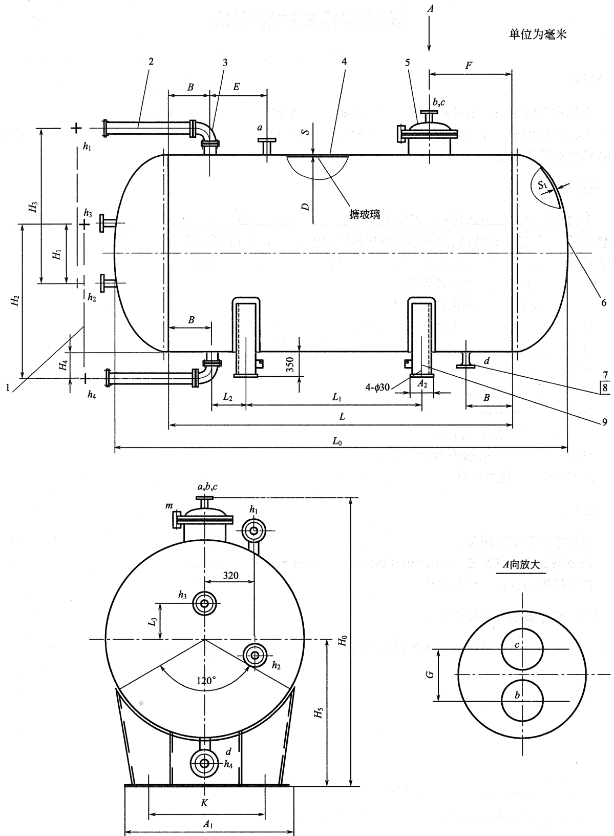
图 1 搪玻璃卧式贮存容器
