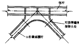
图 8.5.3-2 吊车桁架节点(二)
