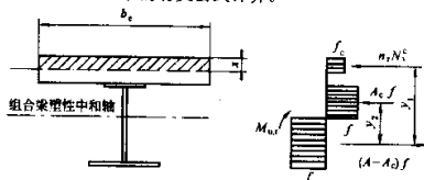
图 11.2.2 部分抗剪连接组合梁计算简图
