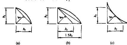
图 7.1.3 直角角焊缝截面
