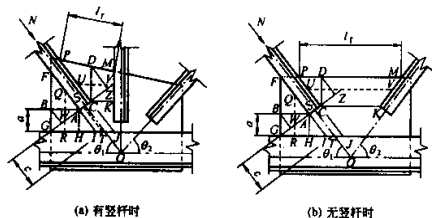
图 F.0.1 节点板稳定计算简图
