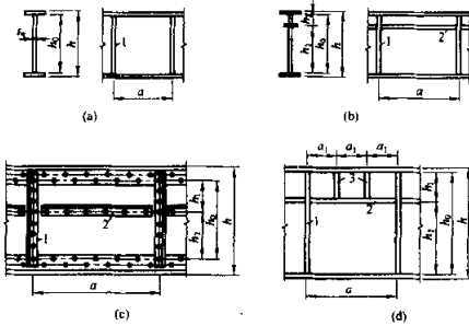
图 4.3.2 加劲肋布置
