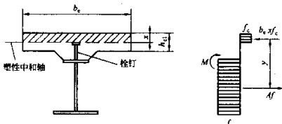
图 11.2.1-1 塑性中和轴在混凝土翼板内的组合梁截面及应力图形
