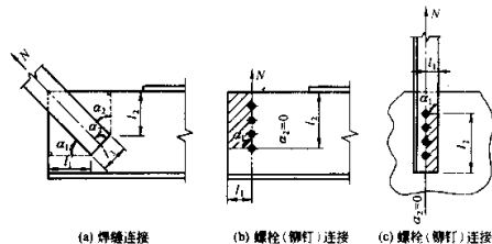
图 7.5.1 板件的拉、剪撕裂
