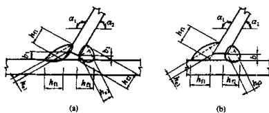
图 7.1.4-2 T 形接头的根部间隙和焊缝截面
