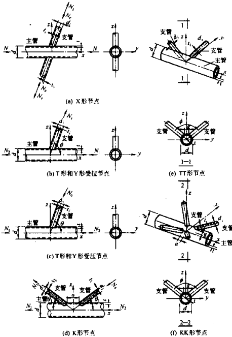
图 10.3.3 圆管结构的节点形式
