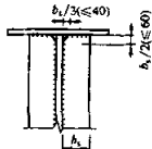
图 8.4.11 加劲肋的切角
