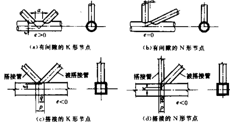
图10.1.5 K形和N形管节点的偏心 and 间隙
