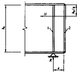
图 4.4.2 设置封头肋的梁端构造
