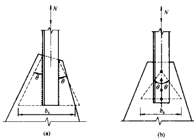
图 7.5.2 板件的有效宽度
