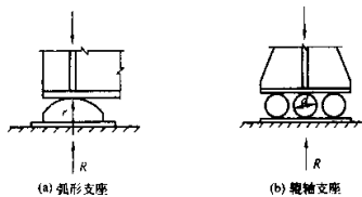
图 7.6.2 弧形支座与辊轴支座示意图
