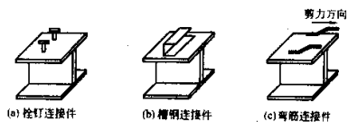
图 11.3.1 连接件的外形及设置方向
