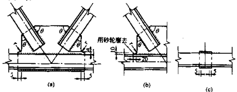
图 8.5.3-1 吊车桁架节点(一)
