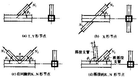
图 10.3.4 矩形管直接焊接水平管节点
