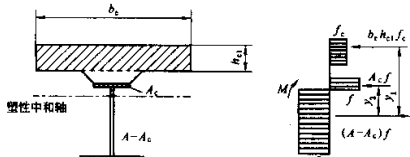
图 11.2.1-2 塑性中和轴在钢梁内的组合梁截面及应力图形
