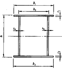
图 4.2.4 箱形截面
