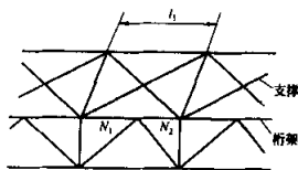
图 5.3.1 弦杆轴心压力在侧向支承点间有变化的桁架简图
